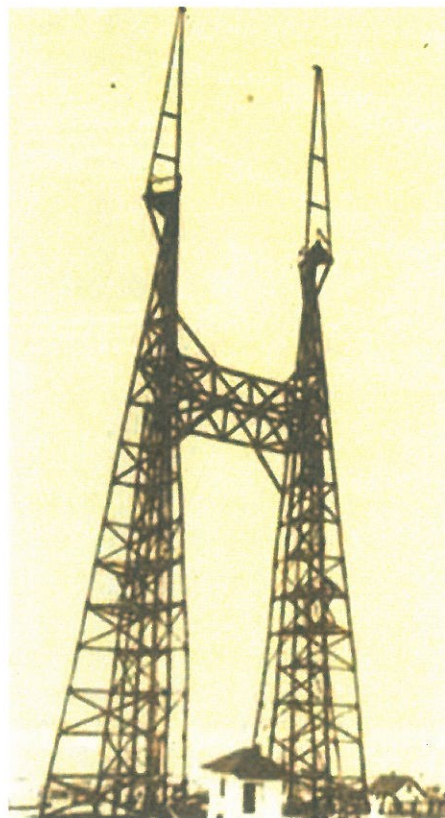
Obr. 1. Murgašov Tón systém (na obrázku je vysielateľ), na ktorý mu bol udelený patent v USA, 10.5.1904.
